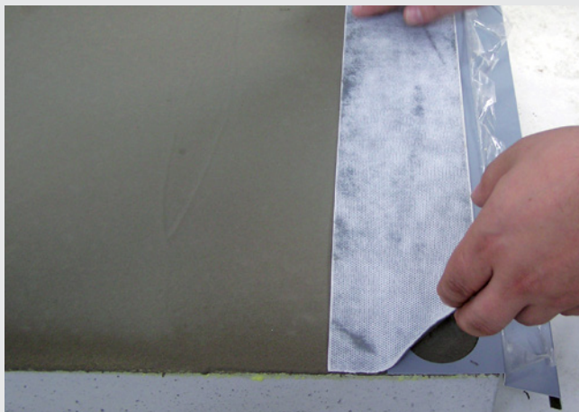
2. Instalarea benzii de etanșare pe balcon la profilul cu picurător marginal
