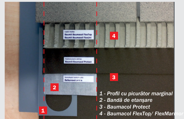
3. Profilul cu picurător marginal trebuie să fie complet acoperit de banda de etanșare!
